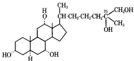
24. 5 \alpha -Bufol
