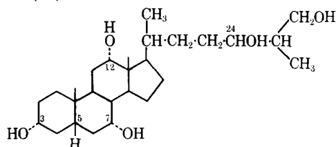
20. Chimaerol
