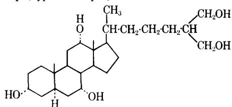
23. 5 \alpha -Cyprinol
