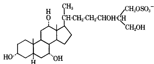
21. Scymnol sulfate
