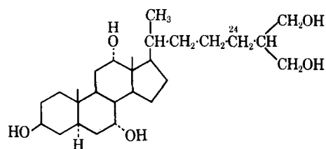
22. Latimerol
